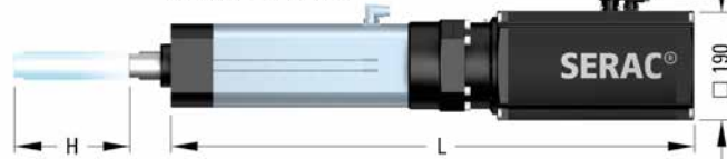
SERAC® LH100-A1
